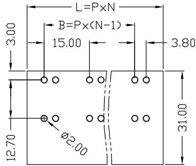
CUTOUT DIMENSIONS
